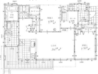
1階平面図
